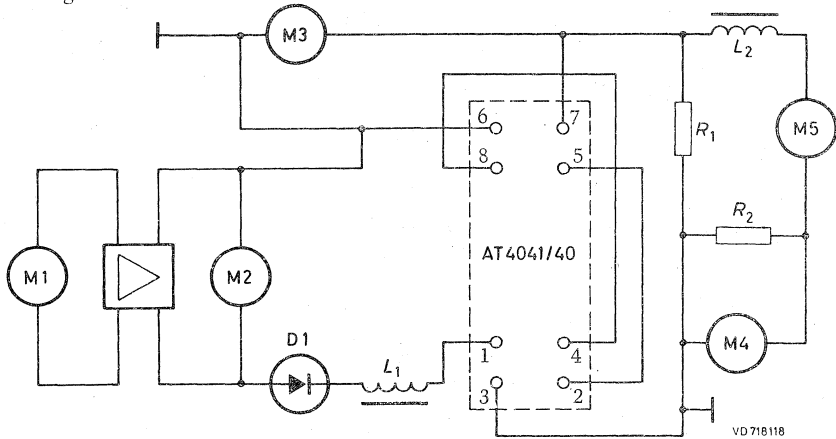
Fig.4 M1 = l.f.generator 3 kHz L1 = 0,7 mH M2 = tube voltmeter L2 = min. 20 mH M3 = oscilloscope D1 = BA148 M4 = tube voltmeter R1 = 10 \Omega , 5 W M5 = l.f.generator 50 Hz R2 = 47 \Omega , 40 W
